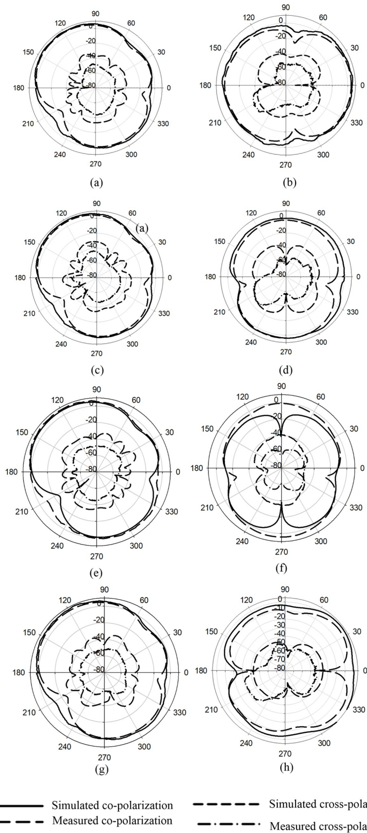
Fig 12. 2D gain pattern at 5.8 GHz (a) Port 1 E-plane (b) Port 1 H-Plane (c) Port 2 E-Plane (d) Port 2 H-Plane (e) Port 3 E-plane (f) Port 3 H-Plane (g) Port 4 E-Plane and (h) Port 4 H-Plane.
