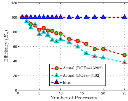
(d) Efficiency
